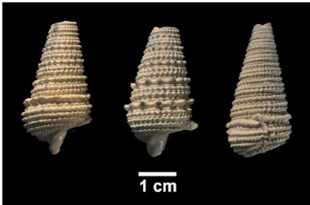
Ukážka variability skulptúry schránok druhu Tympanotonos margaritaceus (BROCCHI)
